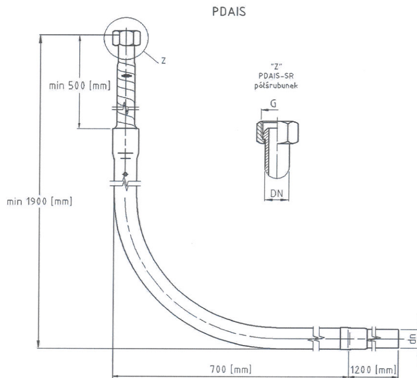
Rys. B12. Polietylenowe przyłącze domowe do gazu kątowe 1x90° z osłoną aluminiową oraz wydłużoną częścią stalową do 0,5 [m] izolowaną taśmą typu: PDAIS-SR.
