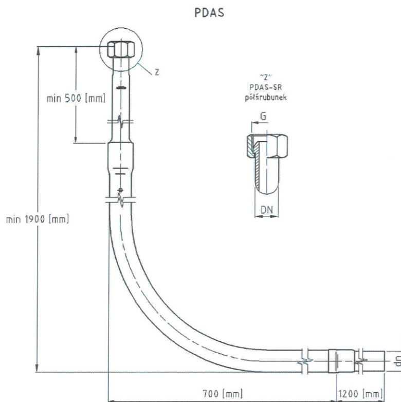
Rys. B13. Polietylenowe przyłącze domowe do gazu kątowe 1x90° z osłoną aluminiową oraz wydłużoną częścią stalową do 0,5 [m] izolowaną cynkową powłoką antykorozyjną, typu: PDAS-SR.
