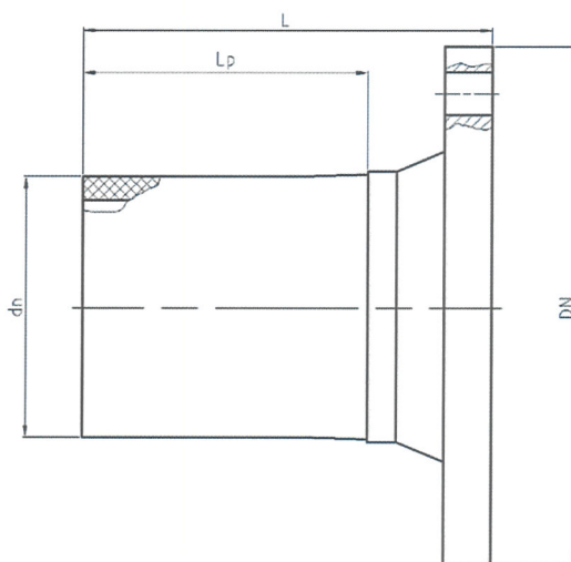
Rys. C2. Połączenie PE/STAL z kołnierzem sztykowym bez spawania dn110 – dn250.
