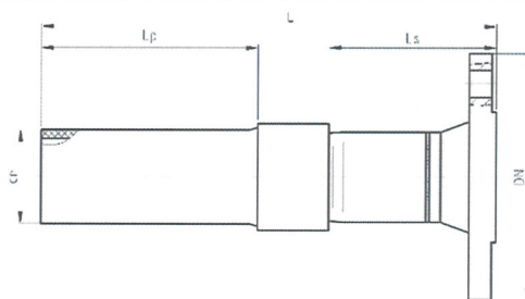
Rys. B1. Połączenie PE/ PE/STAL z kołnierzem szyjkowym.
